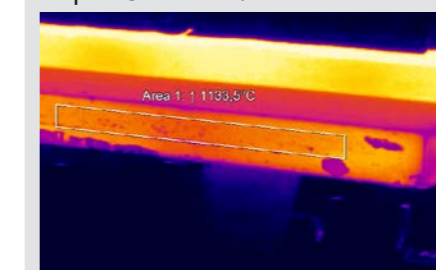
Área de desbordamiento de una planta de fundición continua
