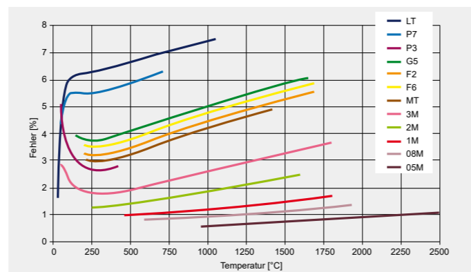
Messfehler bei 10 Prozent falsch eingestelltem Emissionsgrad in Abhängigkeit von der Wellenlänge und Objekttemperatur (LT: 8-14 µm; P7: 7,9 µm; P3: 3,43 µm; G5: 5 µm; MT: 3,9 µm; F2: 4,24 µm; F6: 4,64 µm; 3M: 2,3 µm; 2M: 1,6 µm; 1M: 1,0 µm; 08M: 800nm; 05M: 525 nm)
