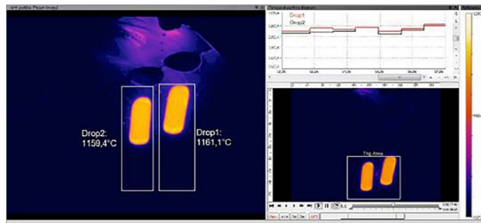
Temperaturüberwachung von geschmolzenen Glaspfropfen mit der Wärmebildkamera PI 1M
