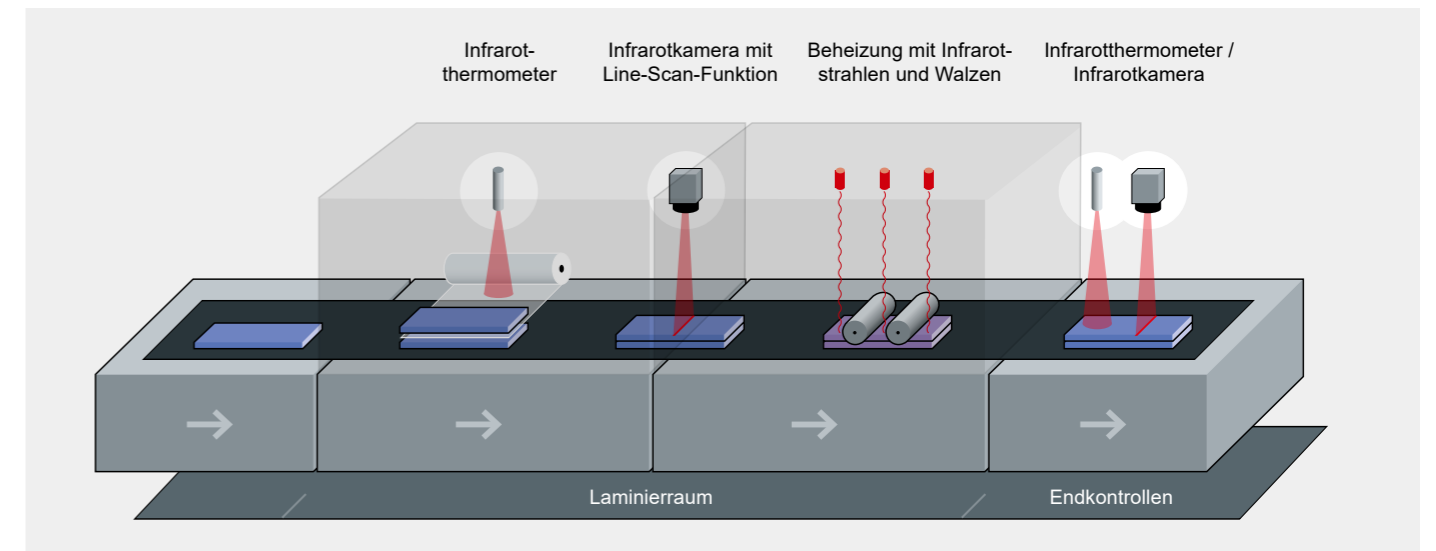
Messbereiche bei der Herstellung von VSG
